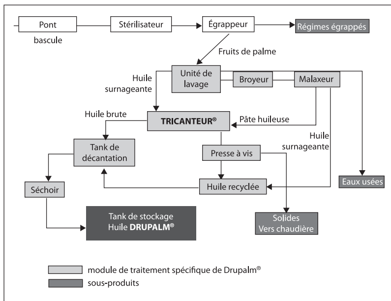
Figure 12.1. Schéma du procédé DRUPALM®.
