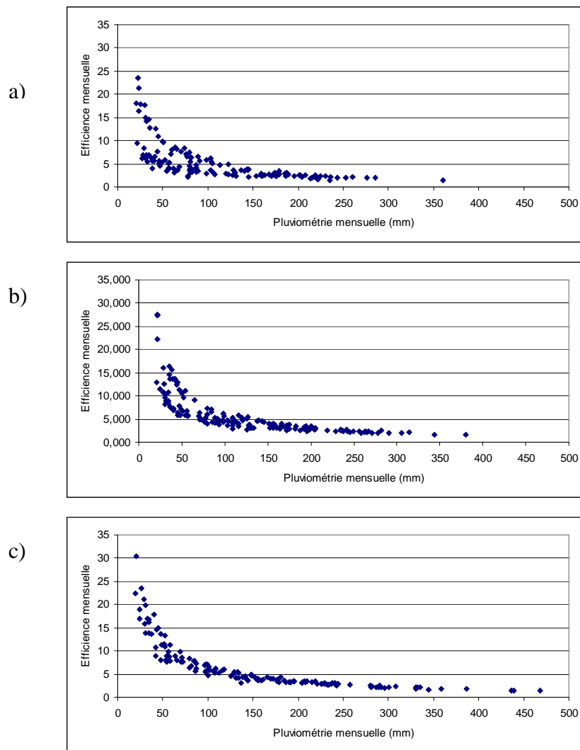
Figure 31 : Efficience pluviométrique mensuelle en fonction des pluies, par paysage : (a) paysage 1 = zone dominée par les cultures. (b) paysage 2 = zone dominée par les savanes ouvertes à fermées. (c) paysage 3 = zone dominée par les savanes arbustives à arborées et les forêts sèches.
