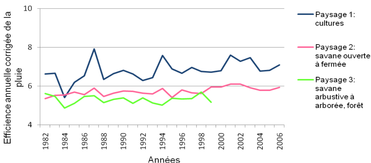
Figure 29 : Efficienc e pluviométrique annuelle normalisée, par paysage.
