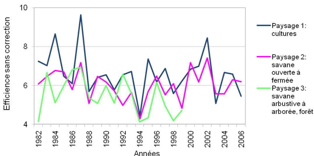
Figure 28 : Efficienc e pluviométrique annuelle, par paysage avant normalisation par la pluie.
