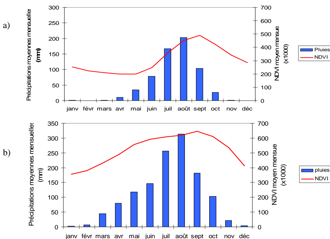
Figure 21 : Variation saisonnière du NDVI et des pluies par sous-bassins. (a) sous-bassin 1 et (b) sous-bassin 7.
