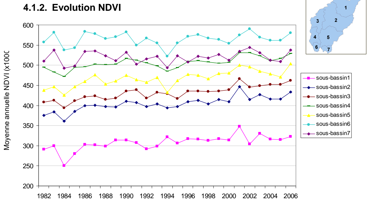
Figure 19 : Evolution du NDVI moyen par sous bassin-versant, moyenne annuelle sur la période 1982-2006
