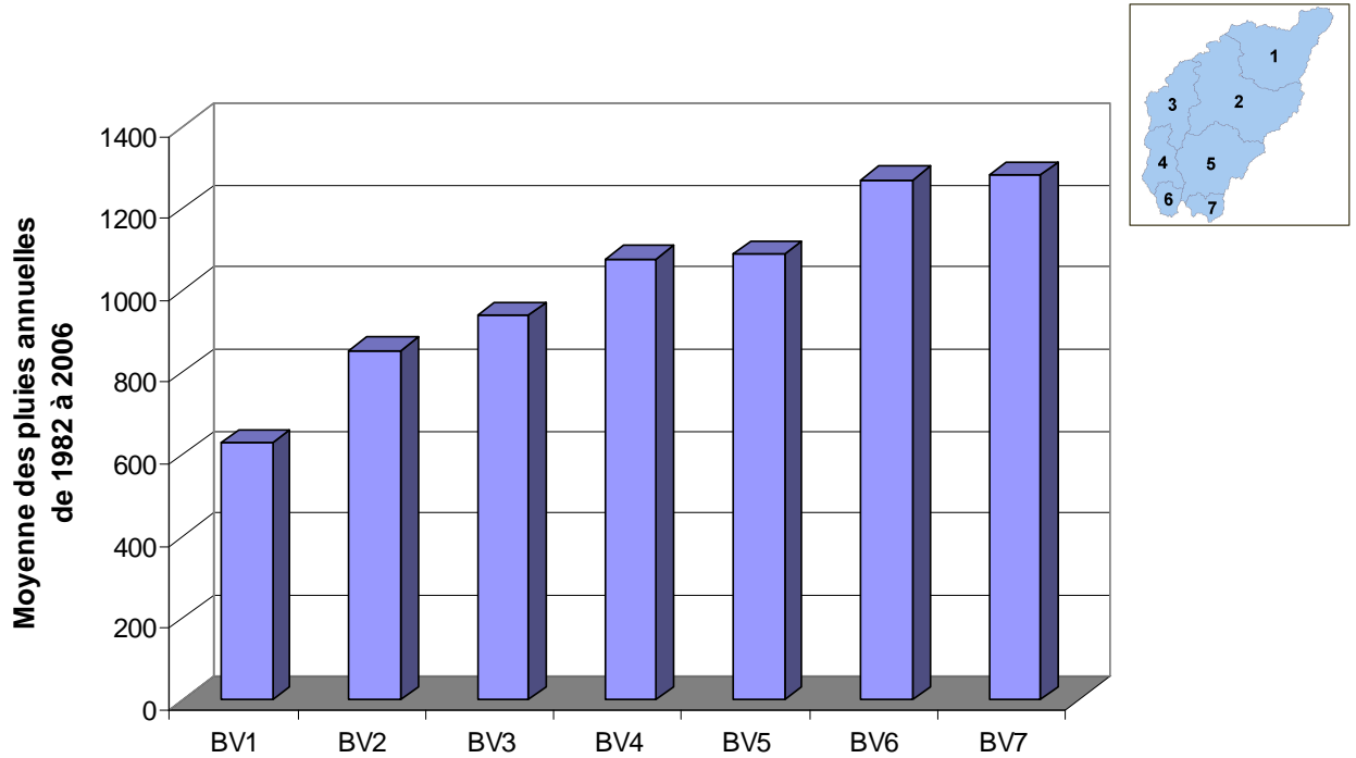
Figure 18 : Pluviométrie annuelle par sous bassins du Bani
