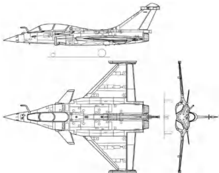
/ “阵风” B 型（双座）战斗机三视图。
