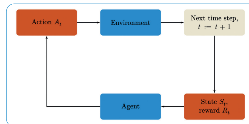
Abb. 1: Der Kreislauf der Interaktion des Agenten mit der Umgebung im Reinforcement Learning. Reinforcement Learning hat aufgrund der Allgemeinheit dieses Konzepts viele Anwendungen. Die Lernalgorithmen berechnen Strategien, denen der Agent bei der Auswahl seiner Aktionen folgt.
