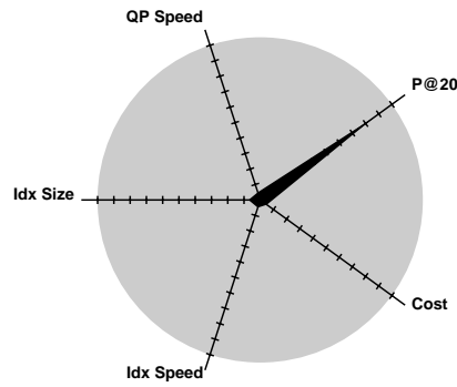
UMass - INQ650
