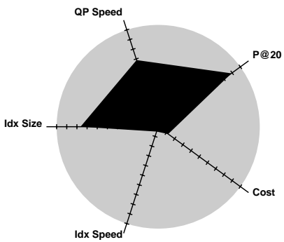
Fujitsu - fl8wlinsb
