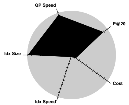
Fujitsu - fl8wlslb
