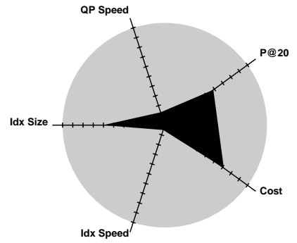
ACSys - acsys8lw0_pr1
