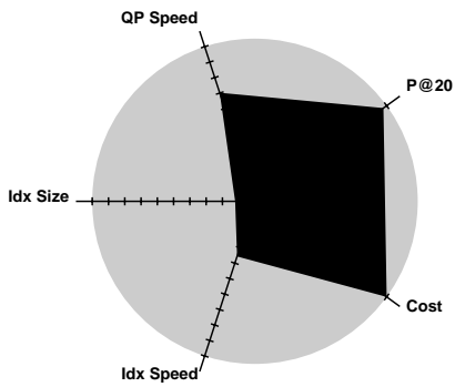
UWaterloo - uwmt8lw1
