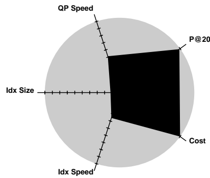
UWaterloo - uwmt8lw2
