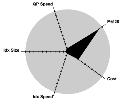
Microsoft - ok8v1
