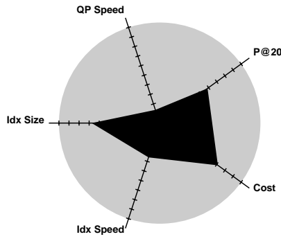
ACSys - acsys8lw0
