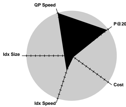
AT&T - att99vlci
