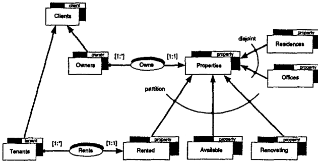
Fig. 1. An Example OM Schema Diagram
